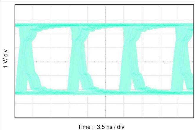
図 9-4. ISO7721 のアイ・ダイアグラム、100Mbps PRBS、5V 電源、25°C
