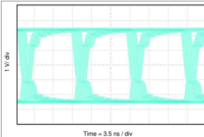
図 9-3. ISO7720 のアイ・ダイアグラム、100Mbps PRBS、5V 電源、25°C
