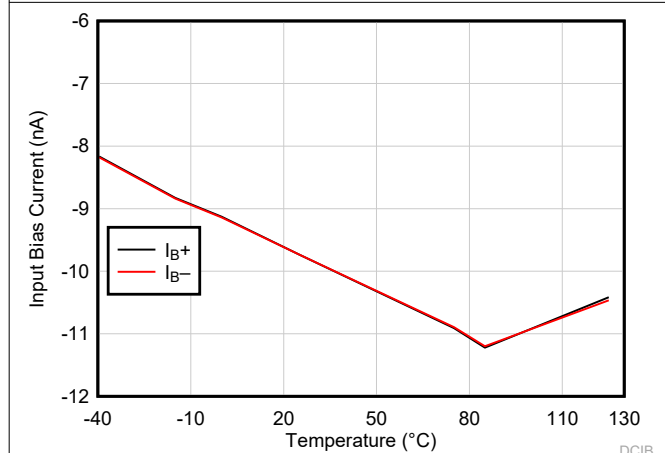
図 6-9. 入力バイアス電流と温度との関係
