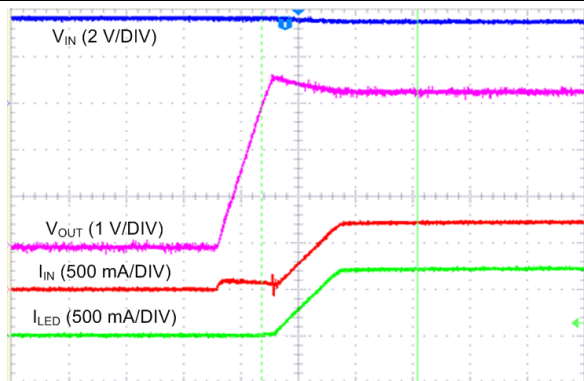
Time (400 \mu\text{s} /DIV) Reg 0x01 = 0xA8
