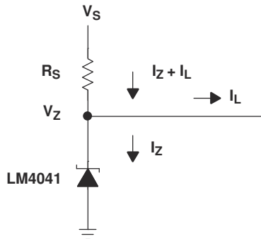
図 7-4. Shunt Regulator
