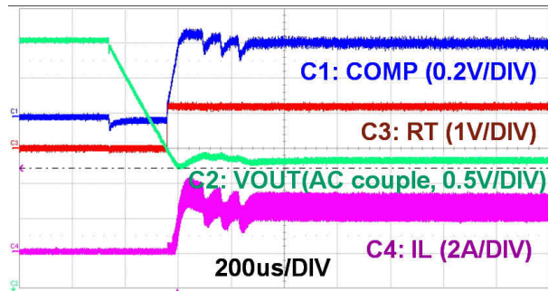
図 9-4. Automatic Wake-Up
