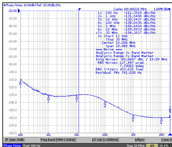
図 8-9. LVDS Phase Noise, 100 MHz
