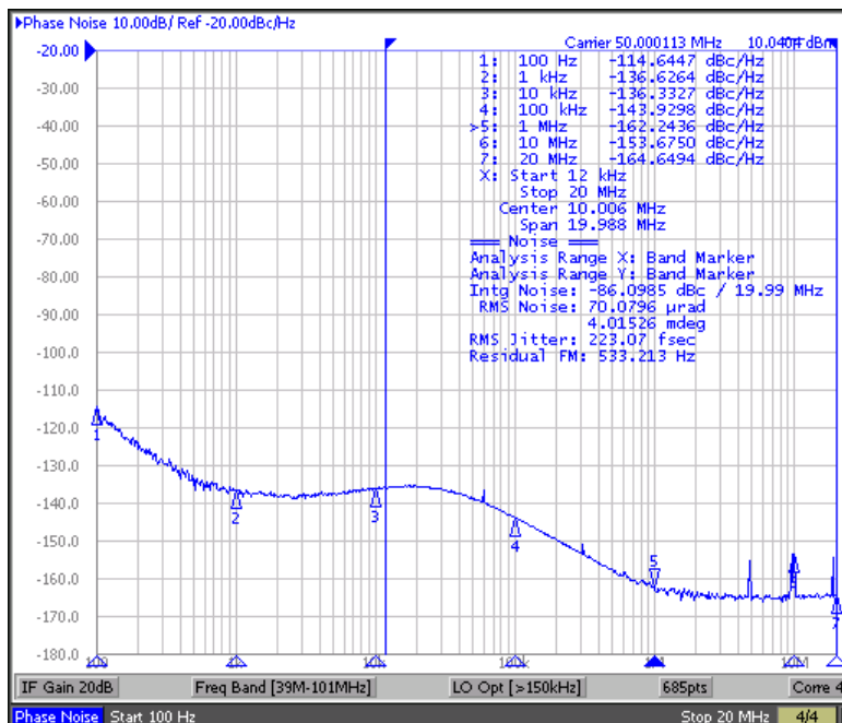
図 8-10. LVCMOS Phase Noise, 50 MHz
