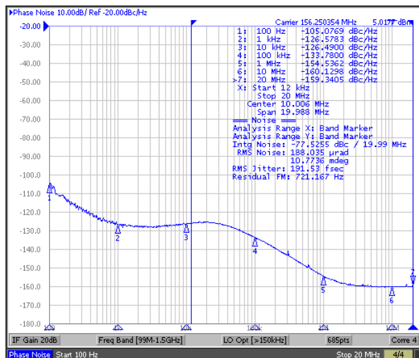
図 8-8. LVPECL Phase Noise, 156.25 MHz
