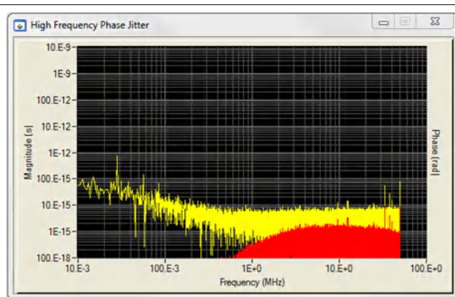
図 8-11. PCIe 3.0 Phase Jitter, 100-MHz HCSL
