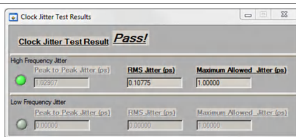
図 8-12. PCIe 3.0 RMS Jitter, 100-MHz HCSL
