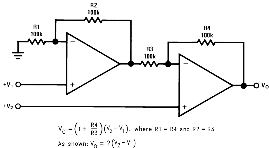
図 9-6.2 オペアンプの計測アンプ
