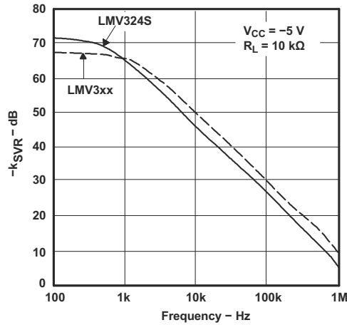
図 6-19. -k_{SVR} と周波数との関係
