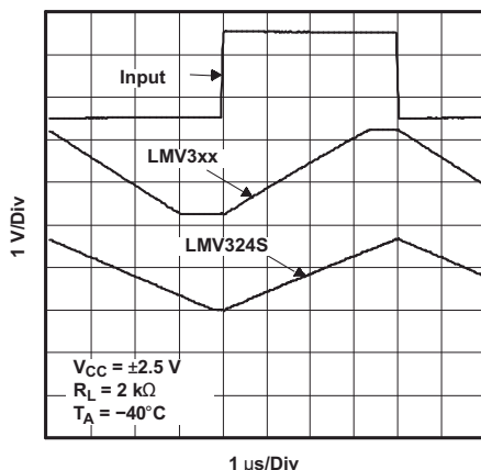
図 6-29. 非反転型の大信号パルス応答
