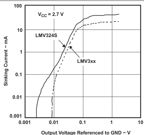
図 6-15. シンク電流と出力電圧との関係
