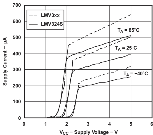
図 6-11. 電源電流と電源電圧との関係：クワッド・アンプ
