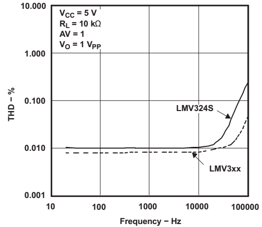
図 6-44. THD + N と周波数との関係
