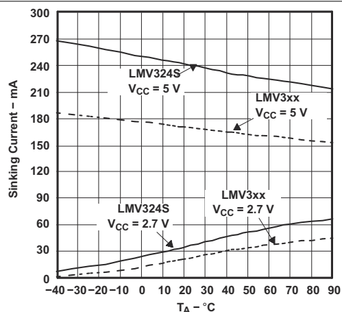
図 6-17. 短絡電流と温度との関係
