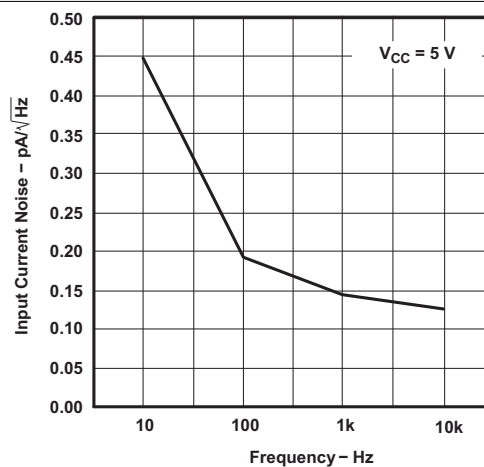
図 6-40. 入力電流ノイズと周波数との関係
