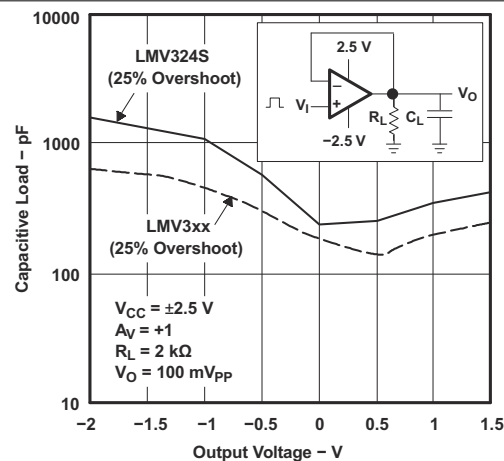
図 6-6. 安定性と容量性負荷との関係
