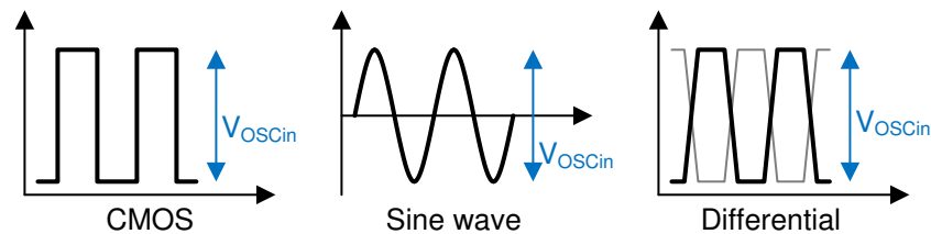
図 164. Input Clock Definition
