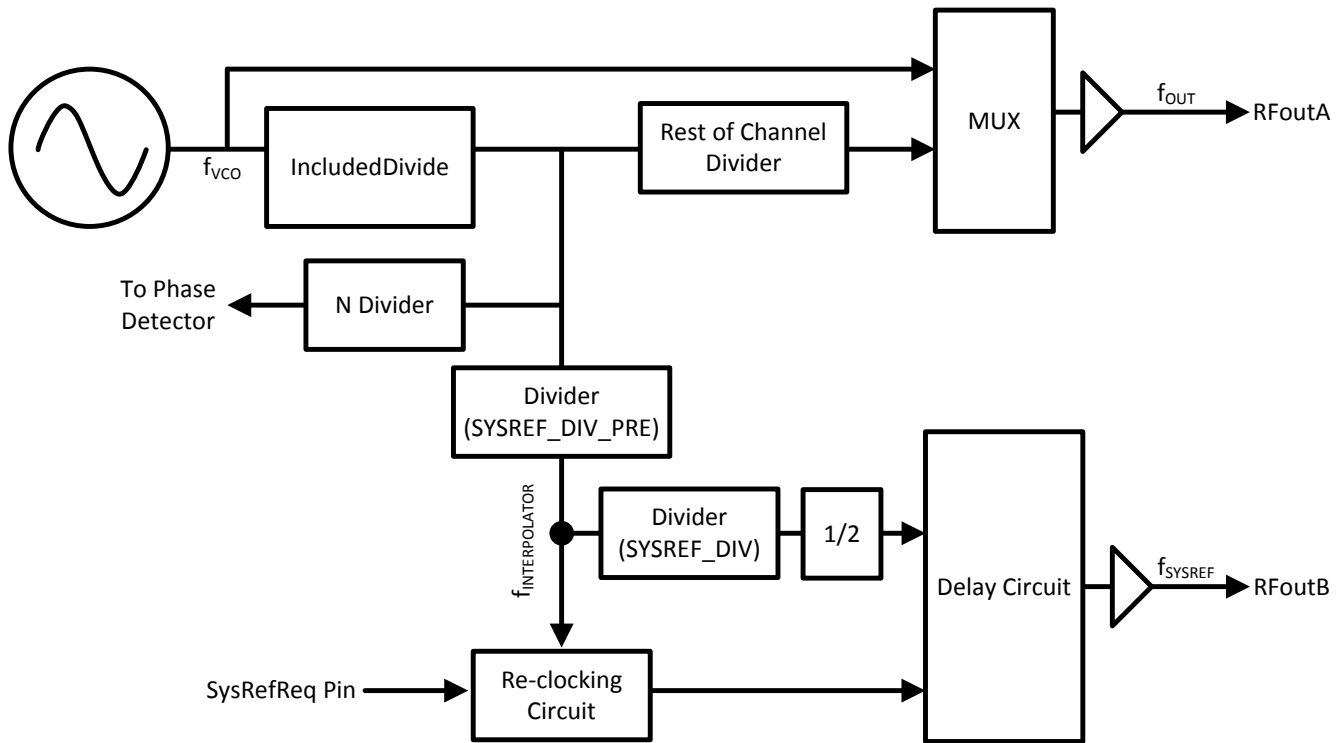
图 27. SYSREF Setup
