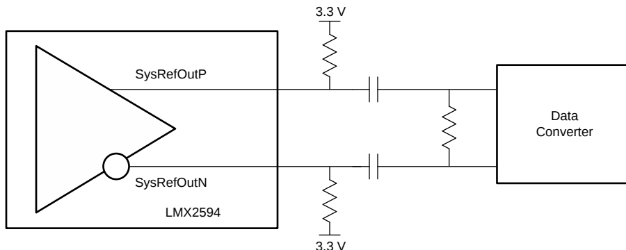
FIG 28. SYSREF Output
