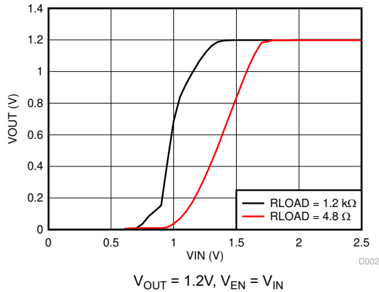
図 5-3. V_{OUT} vs V_{IN}
