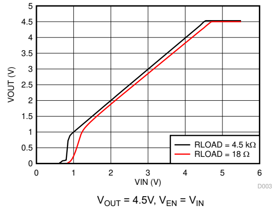
図 5-4. V_{OUT} vs V_{IN}
