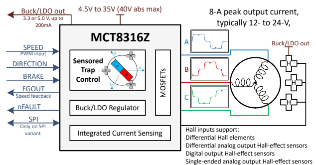
概略回路図
