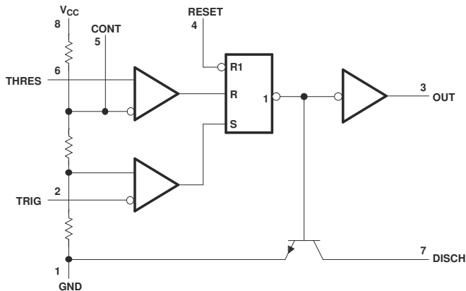
概略回路図
