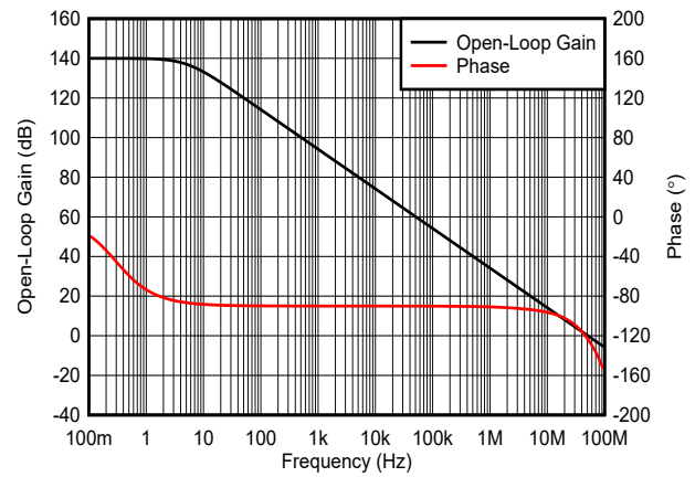
図 6-24. 開ループ・ゲインおよび位相と周波数との関係
