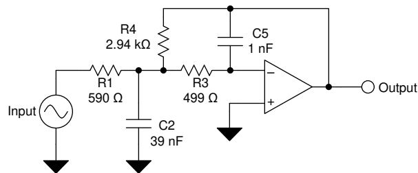
図 8-5. 代表的な OPA828 アプリケーションの回路図
