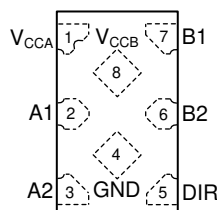
図 4-3. DTM パッケージ、8 ピン X2SON トランスペアレント (上面図)
