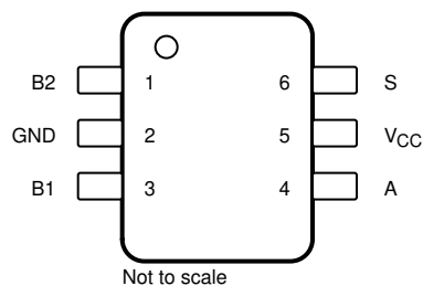
図 4-2. DCK パッケージ、6 ピン SC70 (上面図)
