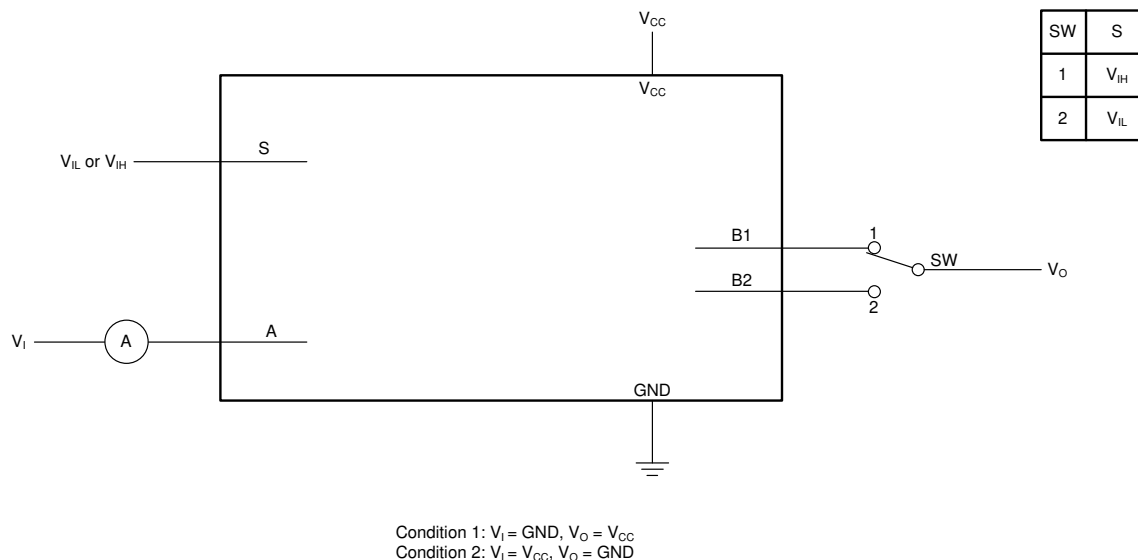
図 13-2. オフ状態スイッチ漏れ電流試験回路
