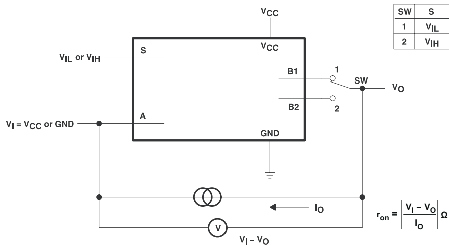
図 13-1. オン状態抵抗試験回路
