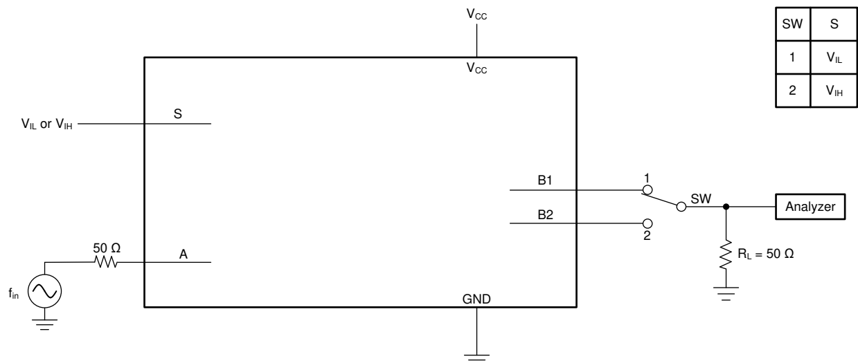
図 13-7. フィードスルー
