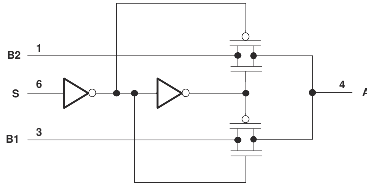
図 14-1. 論理図 (正論理)
