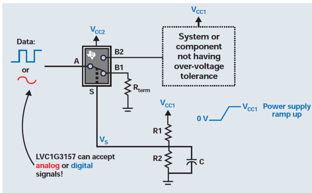
図 15-1. 代表的なアプリケーション回路図
