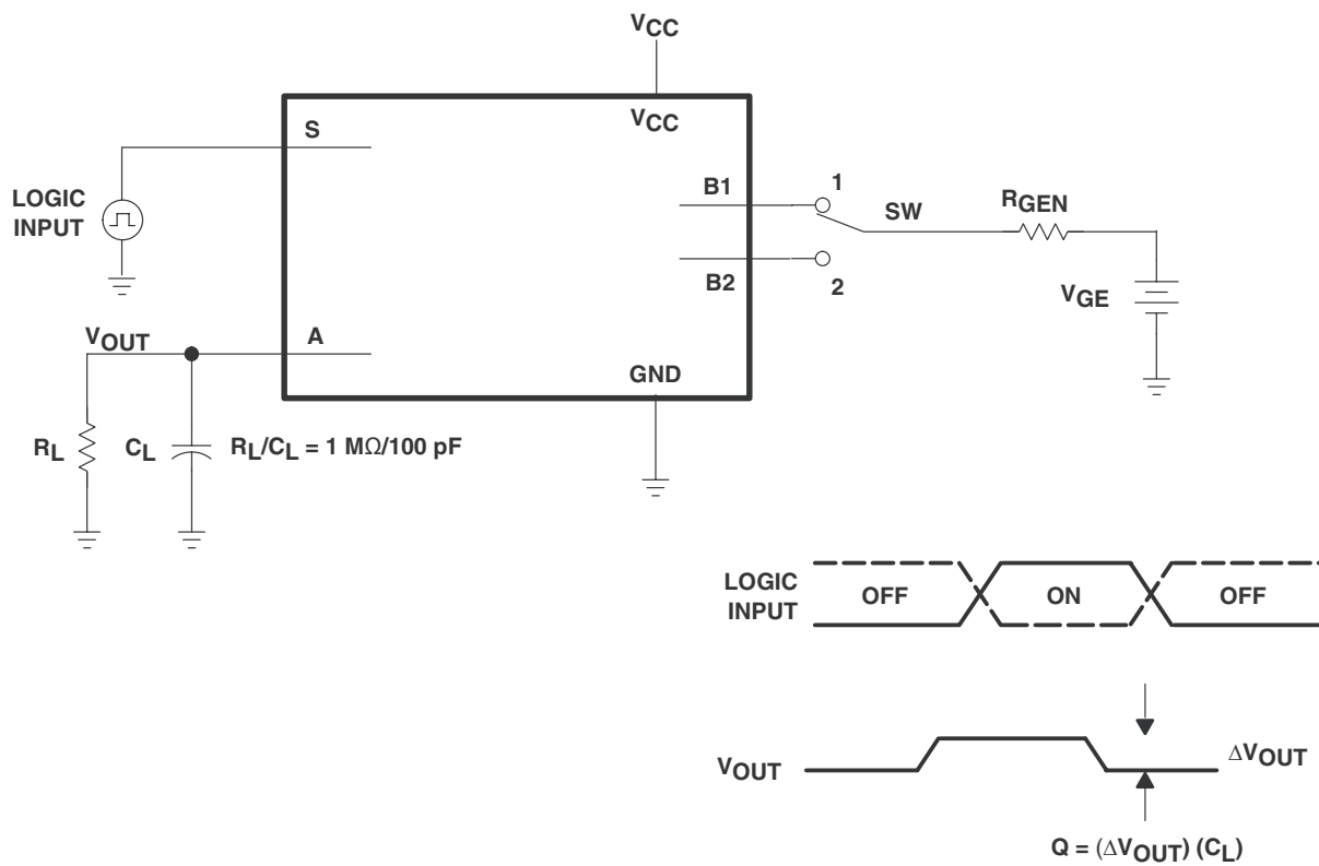
図 13-8. チャージインジェクション試験
