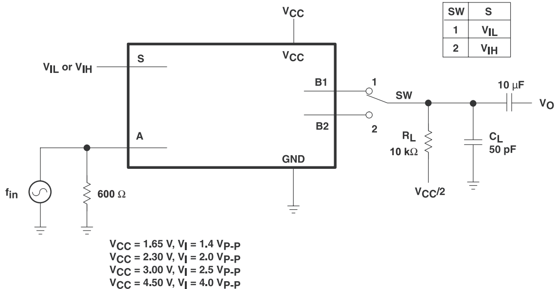
図 13-9. 全高調波歪
