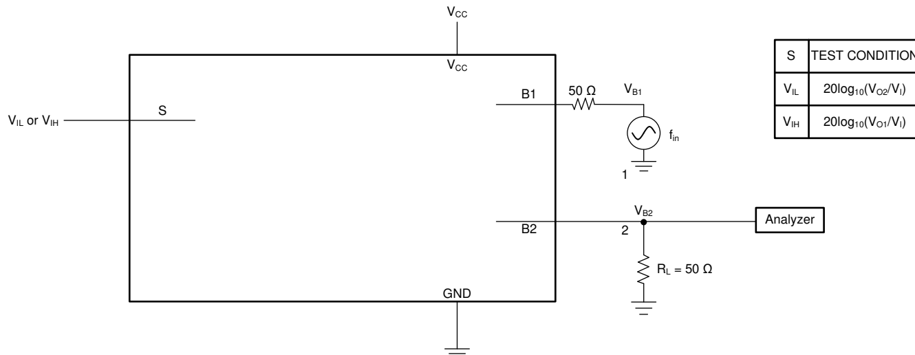
図 13-6. クロストーク (スイッチ間)
