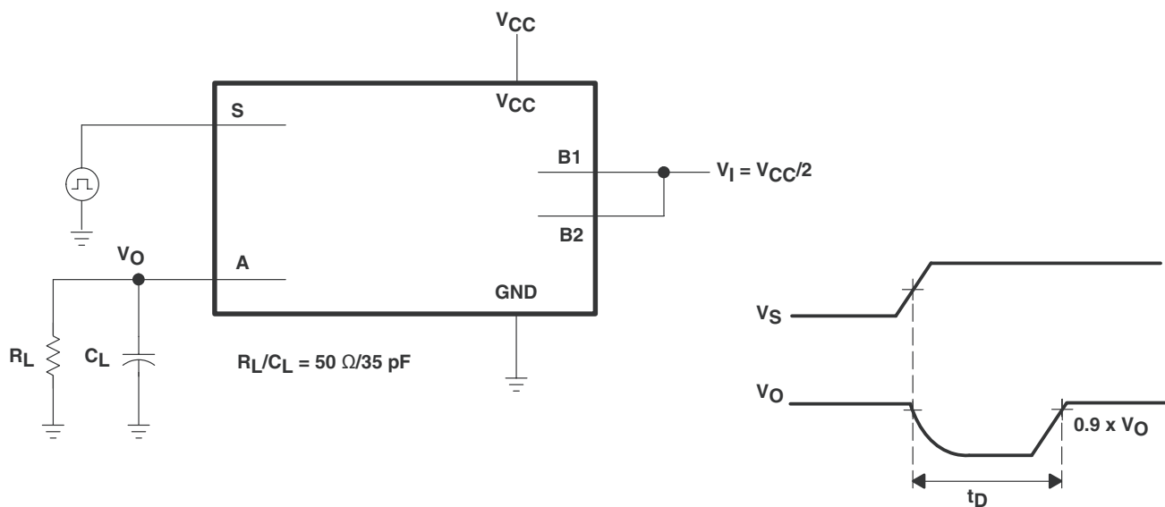
図 13-10. ブレイクビフォーメイク内部タイミング
