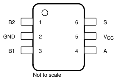
図 4-4. DRL パッケージ、6 ピン SOT (上面図)
