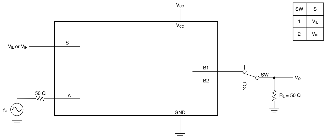
図 13-5. 周波数応答 (スイッチオン時)
