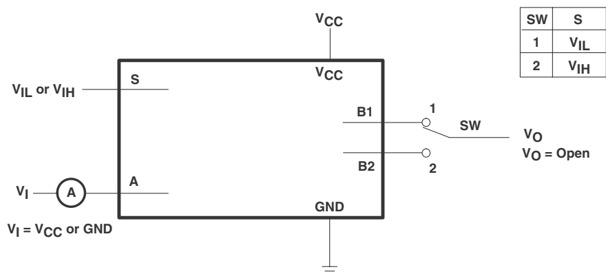
図 13-3. オン状態スイッチ漏れ電流試験回路
