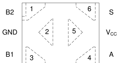
図 4-6. DTB パッケージ、6 ピン X2SON (上面図)
