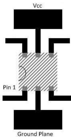
図 17-1. 推奨レイアウト例
