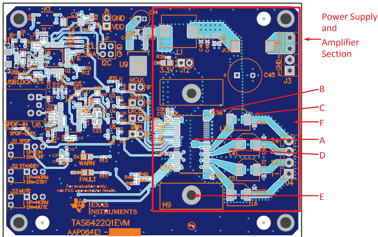
图 80. EVM Layout
