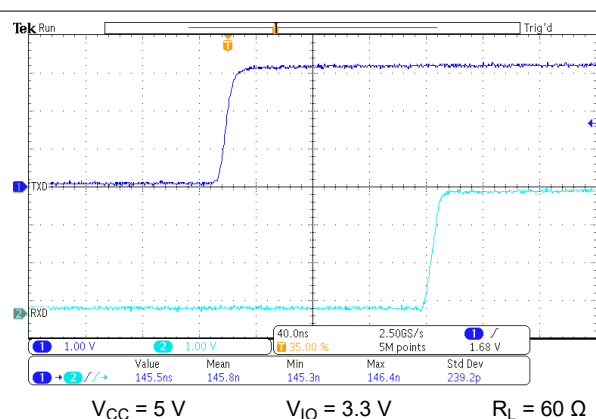
図 8-5. t_{PROP(LOOP2)}
