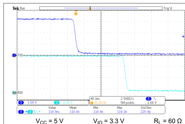
図 8-4. t_{PROP(LOOP1)}
