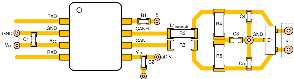
図 8-7. Layout Example
