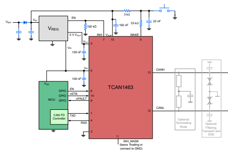
概略回路図
