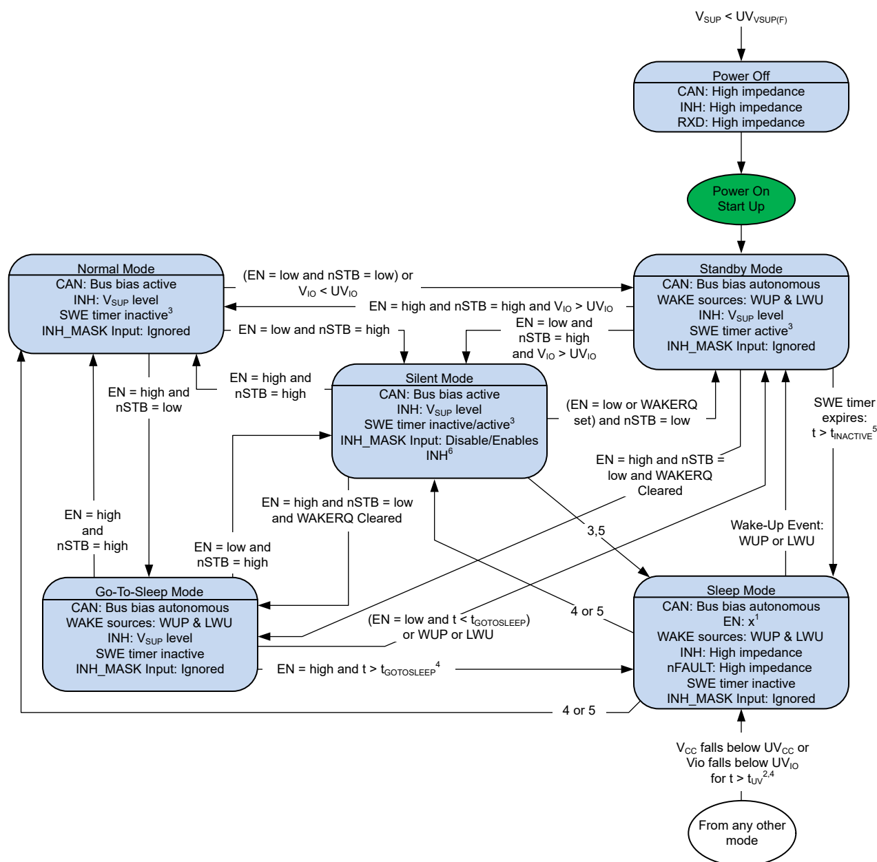
❏ 9-6. TCAN1463-Q1 State Machine
