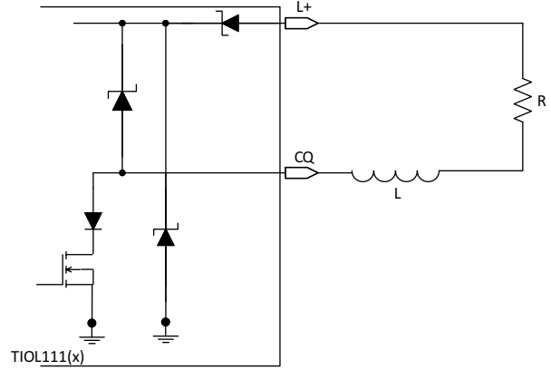
图 19. N-Switch Mode
