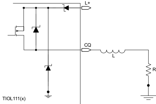
图 18. P-Switch Mode
