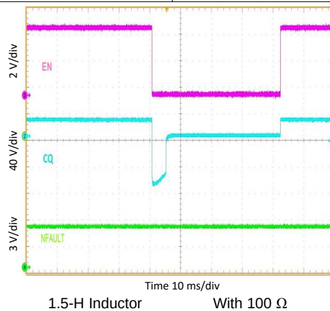
图 30. CQ Driving, High Side Mode
