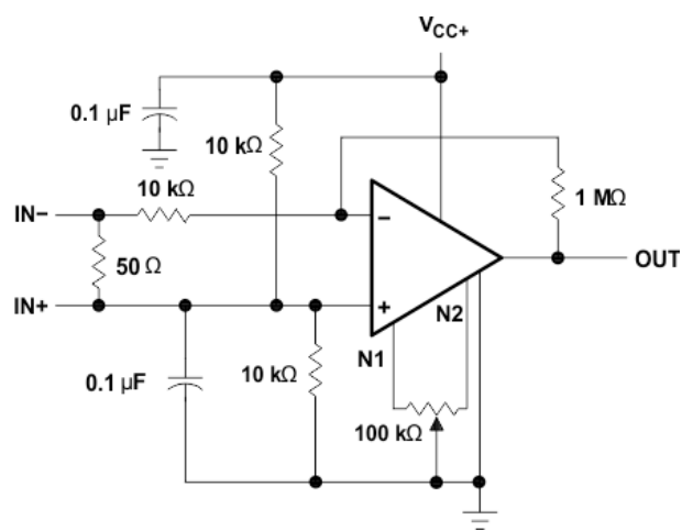
図 9-9. AC アンプ
