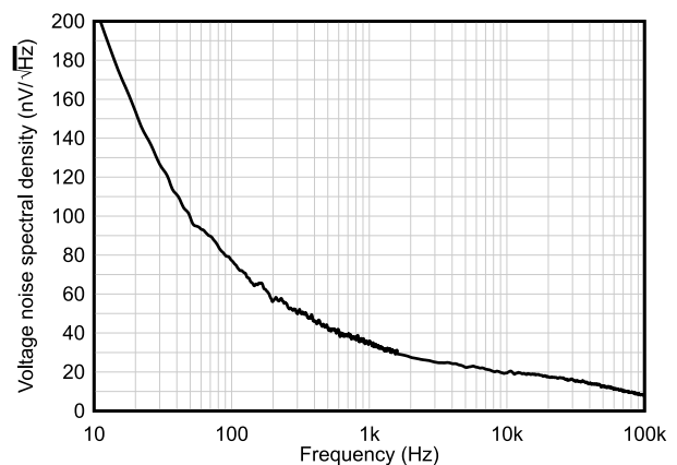
図 6-18. 入力電圧ノイズ・スペクトル密度と周波数との関係
