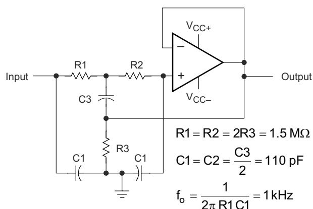
図 9-7. 高 Q ノッチ・フィルタ
