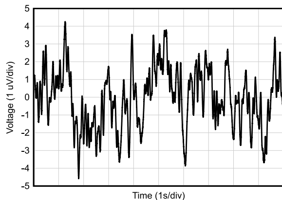
図 6-17. 0.1Hz~10Hz のノイズ
