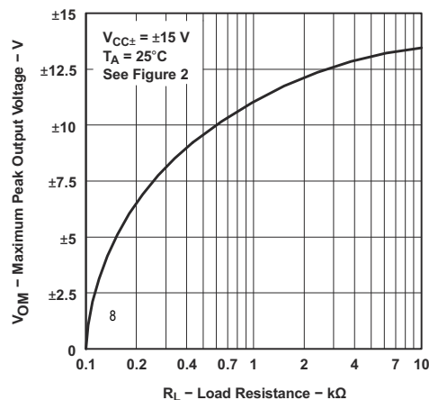
図 6-45. 最大ピーク出力電圧と負荷抵抗との関係
