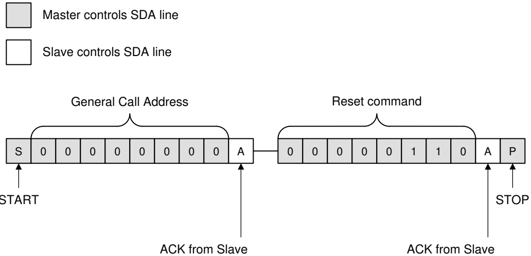
図 7-12. ゼネラル・コール・リセット・コマンドのタイミング図
