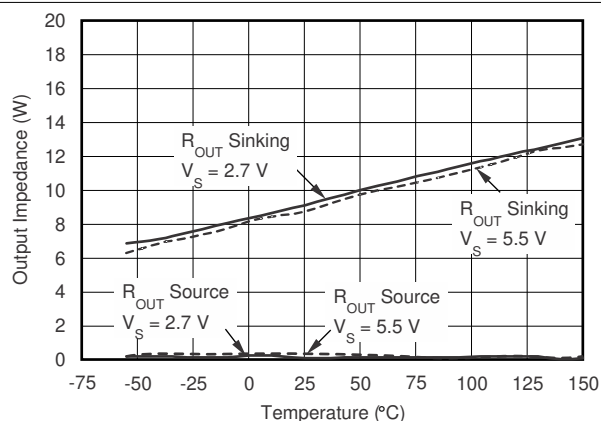
図 6-1. 出力インピーダンスと温度との関係
