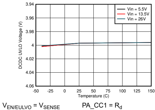
8-7. DCDC UVLO Threshold
