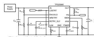
概略回路図
