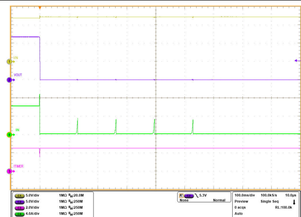
A. 7-29. Circuit Breaker - Auto-Retry
