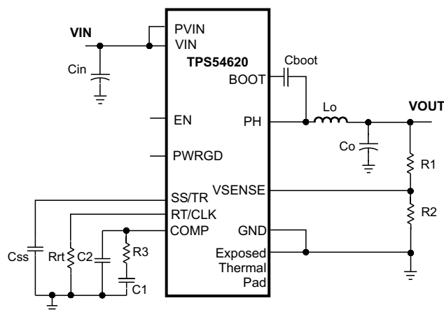
概略回路図
