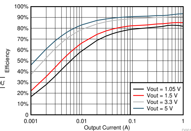
TPS561201 の効率
