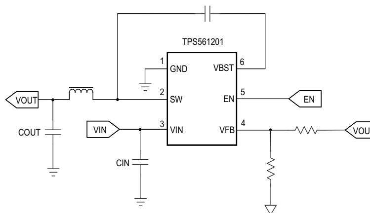
概略回路図
