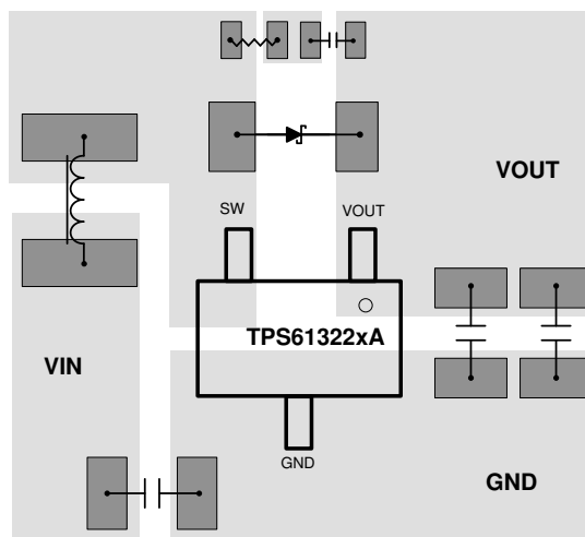
図 10-2. TPS61322xA DBZ Package Layout
