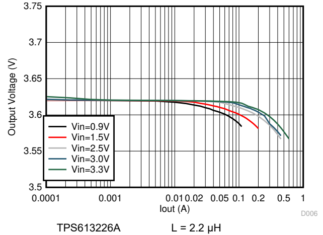
図 6-8. Load Regulation
