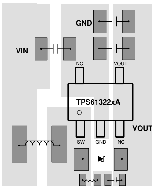
図 10-3. TPS61322xA DBV Package Layout
