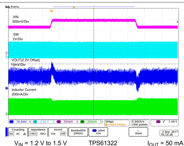
図 8-5. Line Transient
