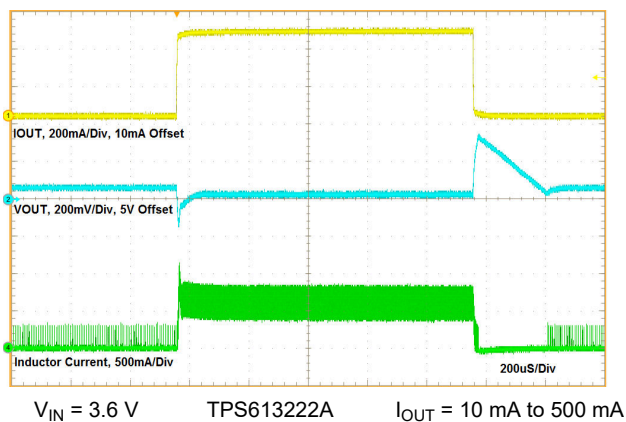
図 8-16. Load Transient
