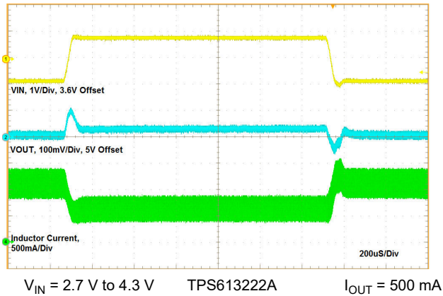
図 8-14. Line Transient
