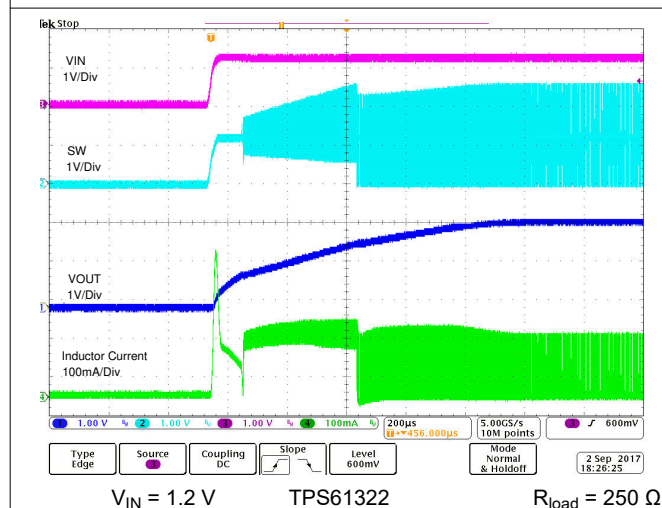
図 8-4. Start-up by VIN
