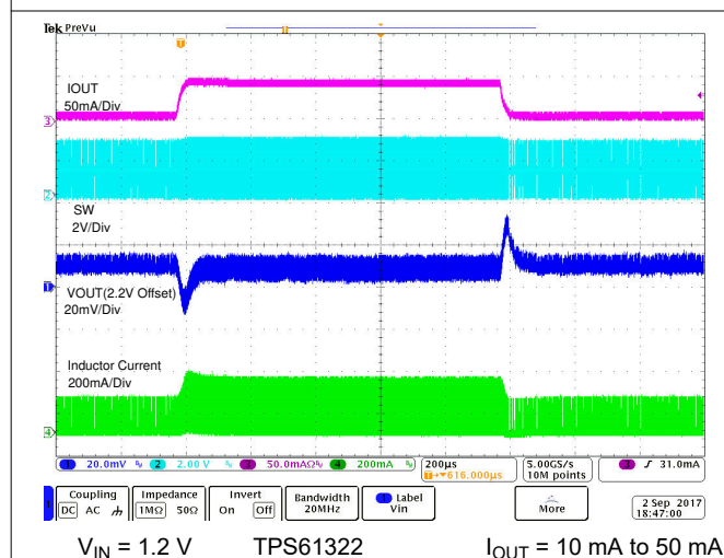
図 8-6. Load Transient
