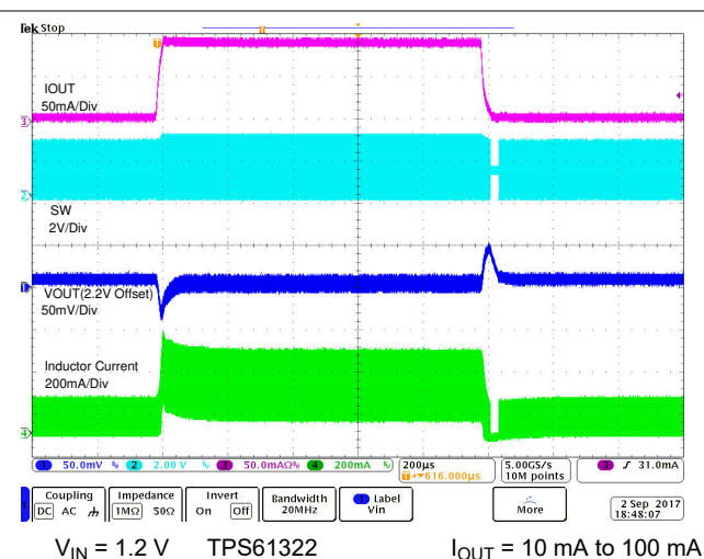
図 8-7. Load Transient
