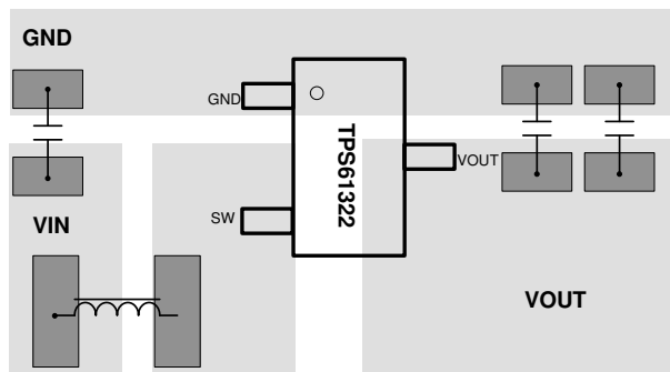
図 10-1. TPS61322 Layout
