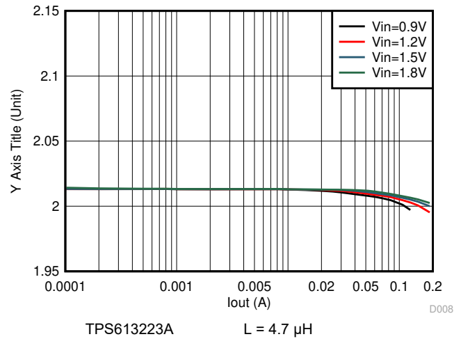
図 6-10. Load Regulation
