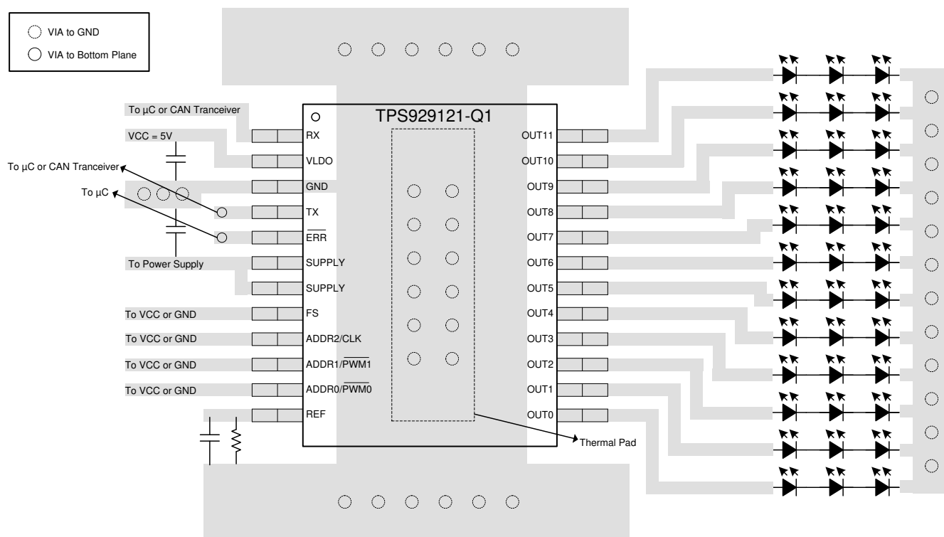
11-1. TPS929121-Q1 Layout
