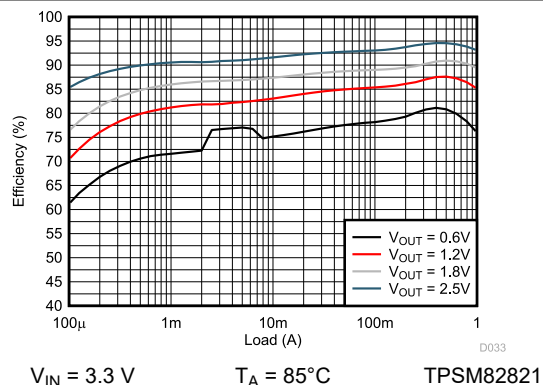
图 9-8. Efficiency
