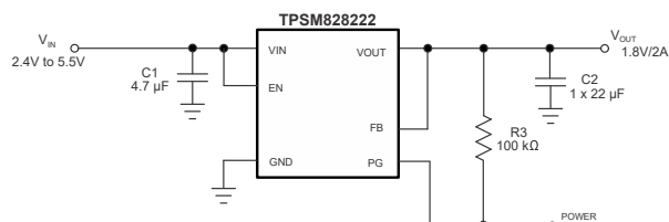
1.8V の出力電圧に設定された固定出力アプリケーション
