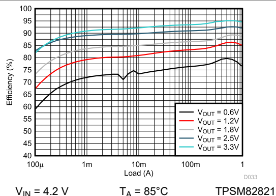
图 9-6. Efficiency
