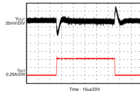
图 9-26. Load Transient
