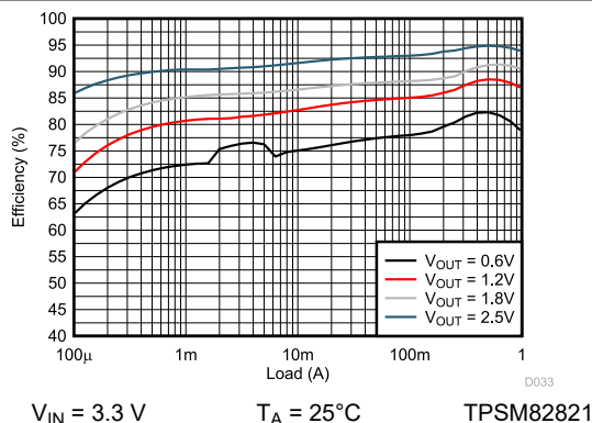
图 9-7. Efficiency
