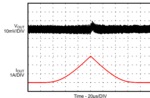
9-156. Load Sweep
