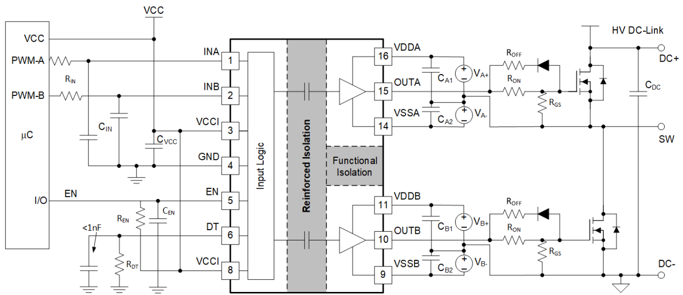
図 8-1. デュアル電源を使用した代表的なアプリケーションの回路図
