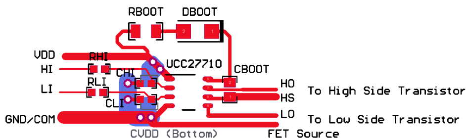
✎ 53. UCC27710 Layout Example
