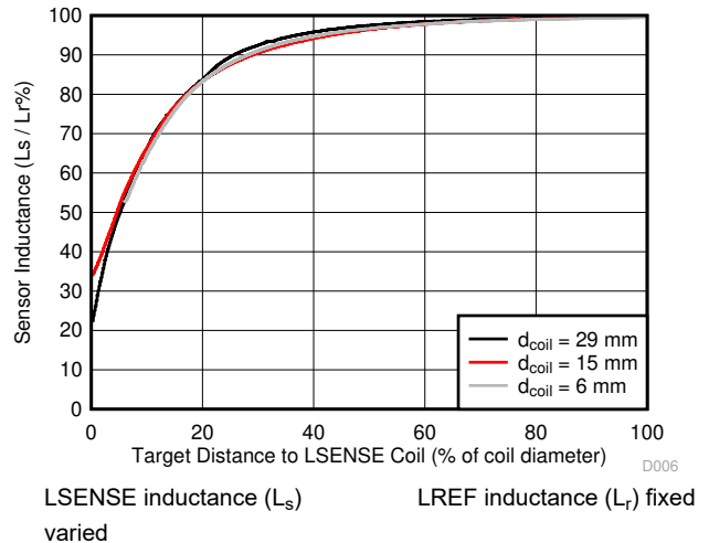
図 5-6. Inductance vs. Distance
