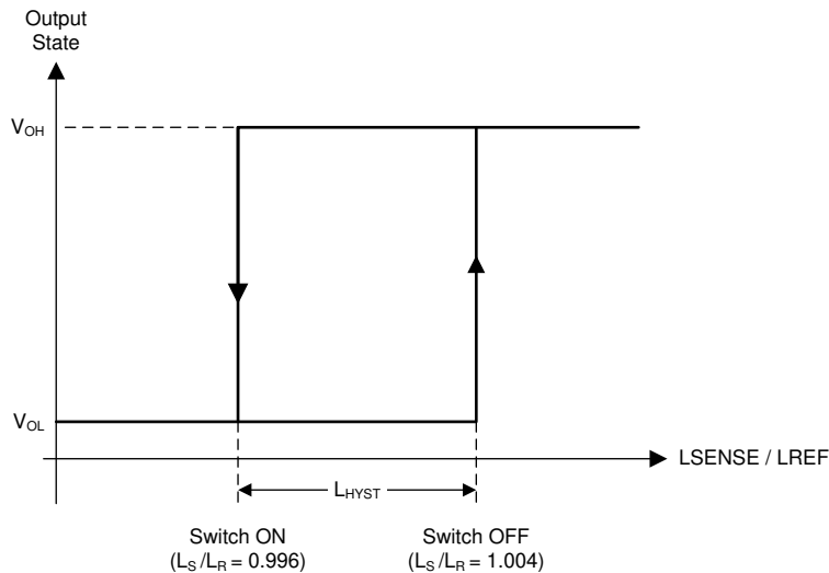
図 6-6. Inductance Hysteresis
