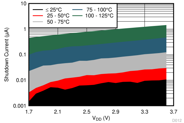
図 5-12. I_{\text{SD}} vs. V_{\text{DD}}
