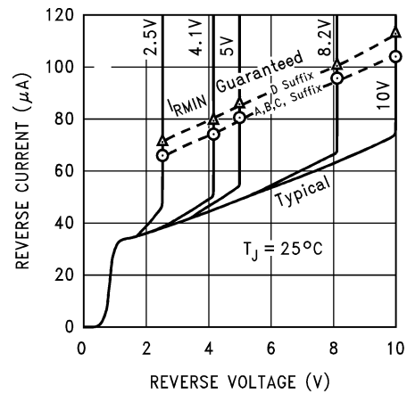
図 5-4. 逆特性と最小動作電圧
