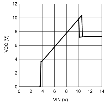
FIG 5-22. VCC vs VIN
