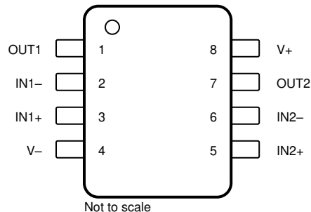
図 7-4. TLV9062-Q1、D、DGK、PW パッケージ 8 ピン SOIC、VSSOP、TSSOP (上面図)
