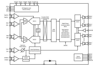
ADC12DJ4000RF ブロック図
