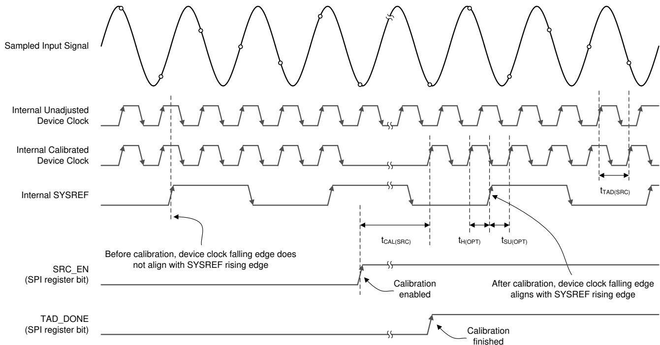
图 8-3. SYSREF Calibration Timing Diagram
