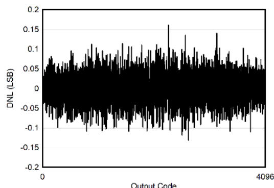
7-6. DNL vs ADC Code
