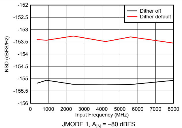
图 6-36. DES Mode: NSD vs Input Frequency
