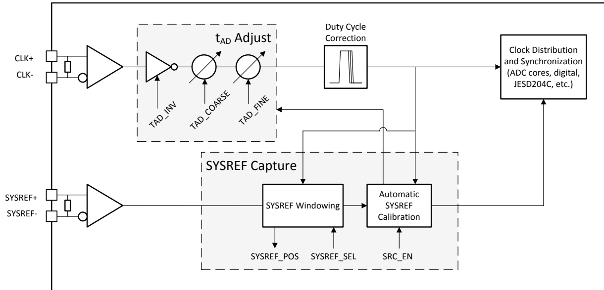
图 6-2. Clocking Subsystem
