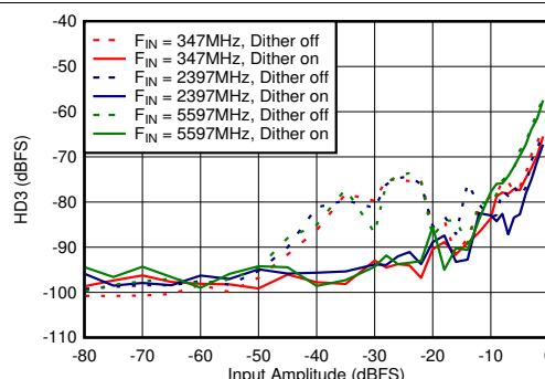
图 6-66. DES Mode: HD3 vs Input Amplitude and Dither
