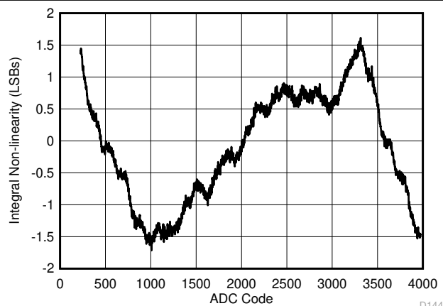
图 6-4. INL vs ADC Code
