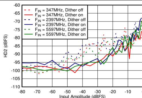
图 6-64. DES Mode: HD2 vs Input Amplitude and Dither
