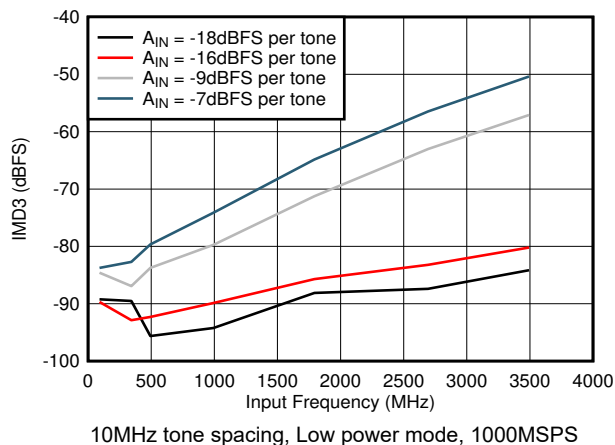
7-76. IMD3 vs F_{IN}
