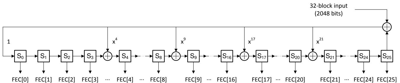
図 8-8. FEC Parity Bit Generator
