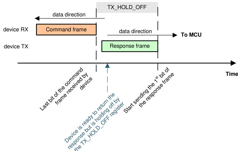
図 8-25. UART TX_HOLD_OFF
