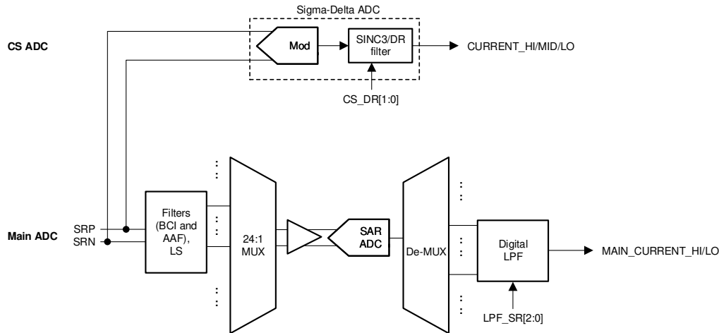
図 8-12. CS ADC
