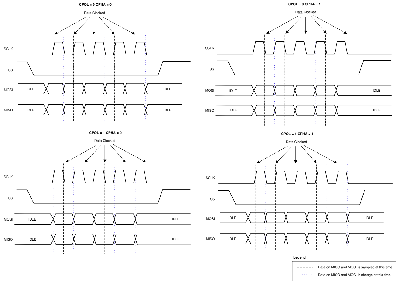
図 8-28. SPI Controller CPOL and CPHA
