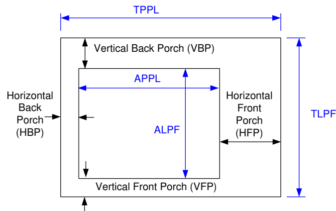
FIG 11-1. Parameter Definitions
