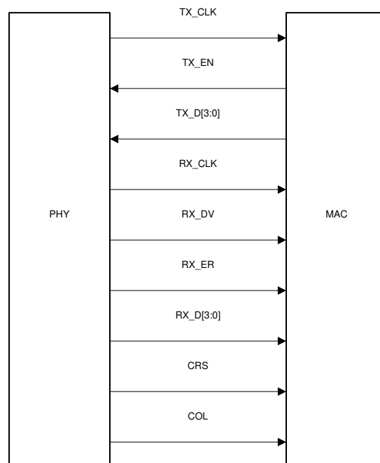
図 8-4. MII Signaling
