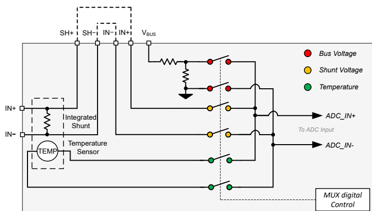
图 7-3. High-Voltage Input Multiplexer
