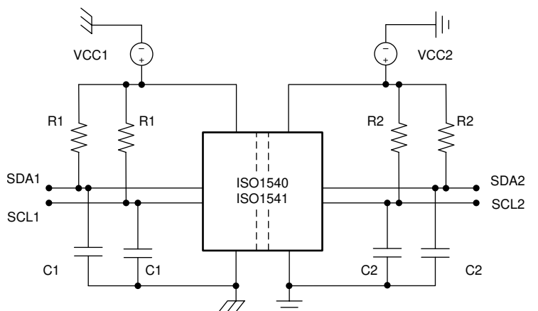
图 7-1. Test Diagram
