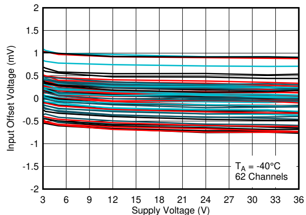
図 5-11. -40°Cでの入力オフセット電圧と電源電圧との関係
