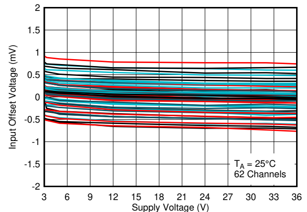
図 5-12. 25°Cでの入力オフセット電圧と電源電圧との関係
