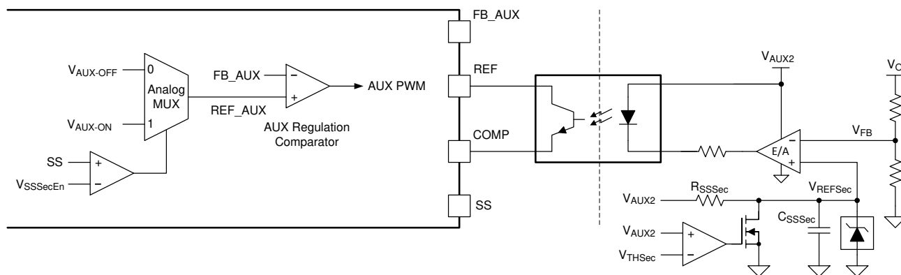
图 7-8. Soft-Start Function
