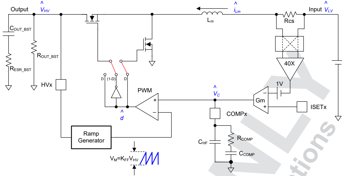
图 8-3. Boost Loop Block Diagram
