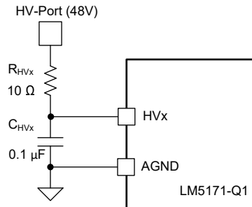
8-9. HVx Pin Configuration
