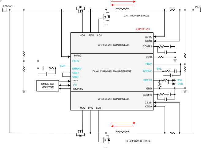
アプリケーションの簡略回路図
