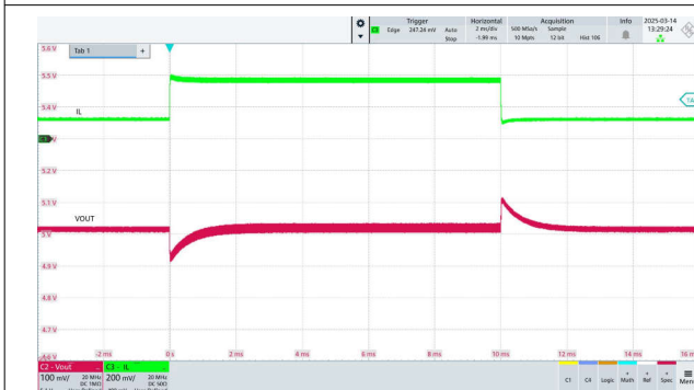
図 7-10. Load Regulation
