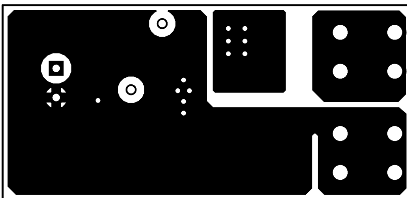
図 7-13. Solder Side
